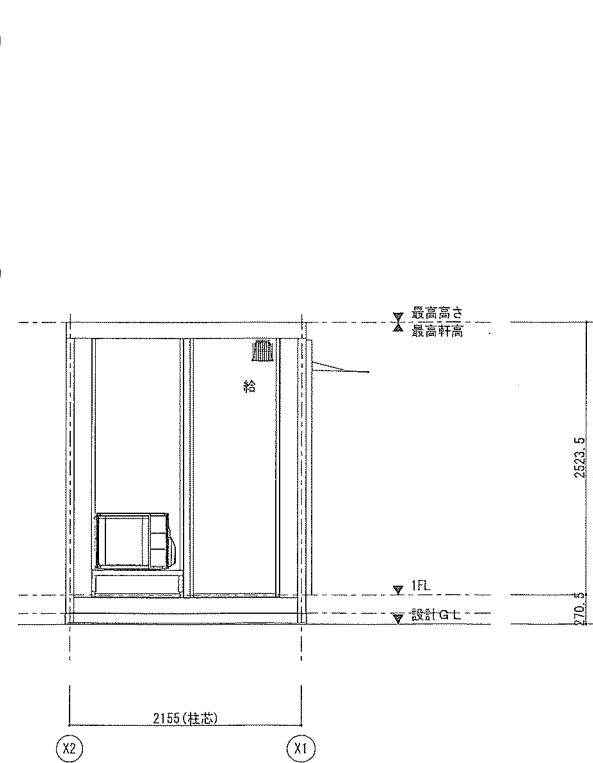
Y2通り立面図
