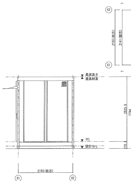
Y1通り立面図
