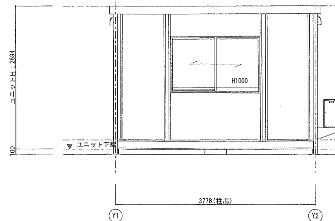
X2通り立面図
