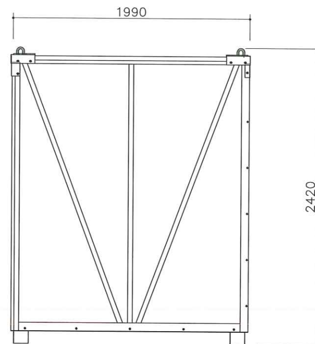
X1通り立面図
