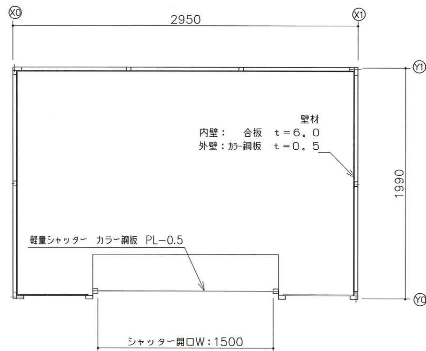
平面図
