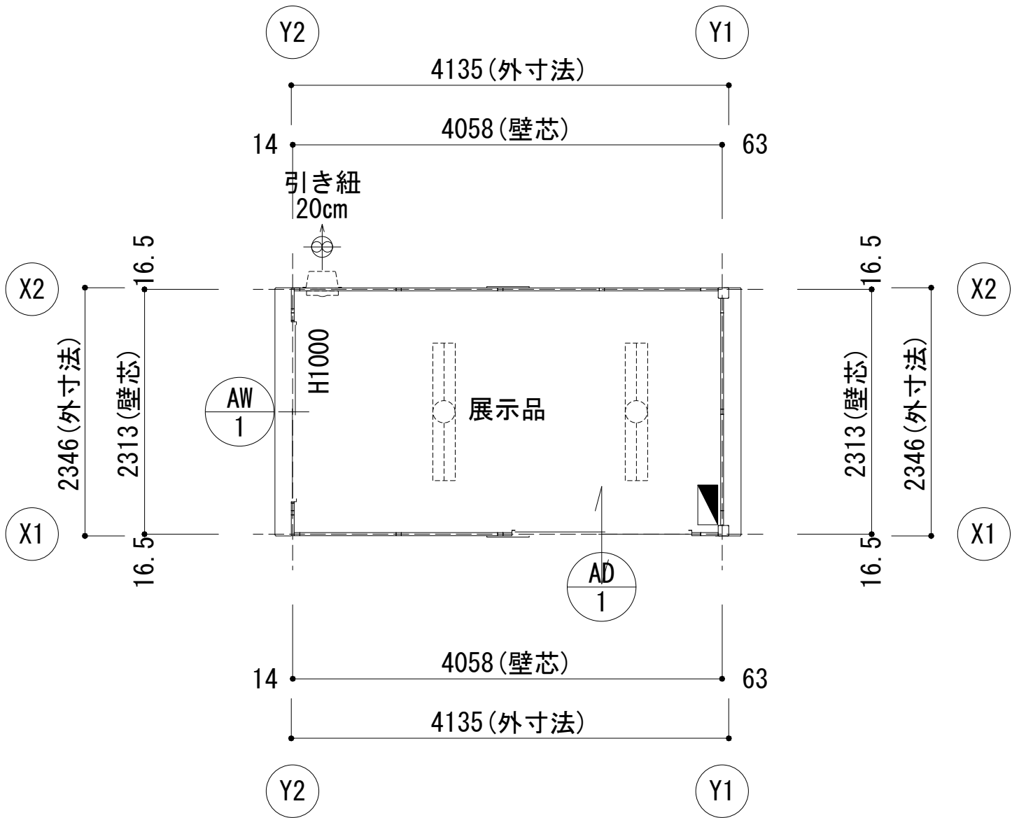
1階平面図
