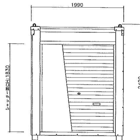
X1-X2 通り立面図
