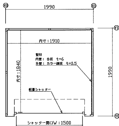
平面図
