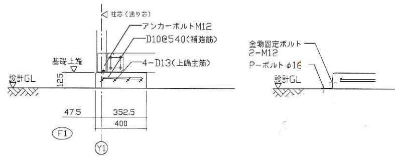
基礎断面図 S=1:20
