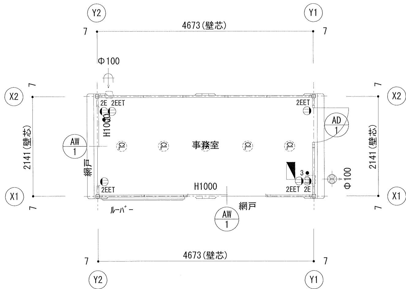
1階平面図
