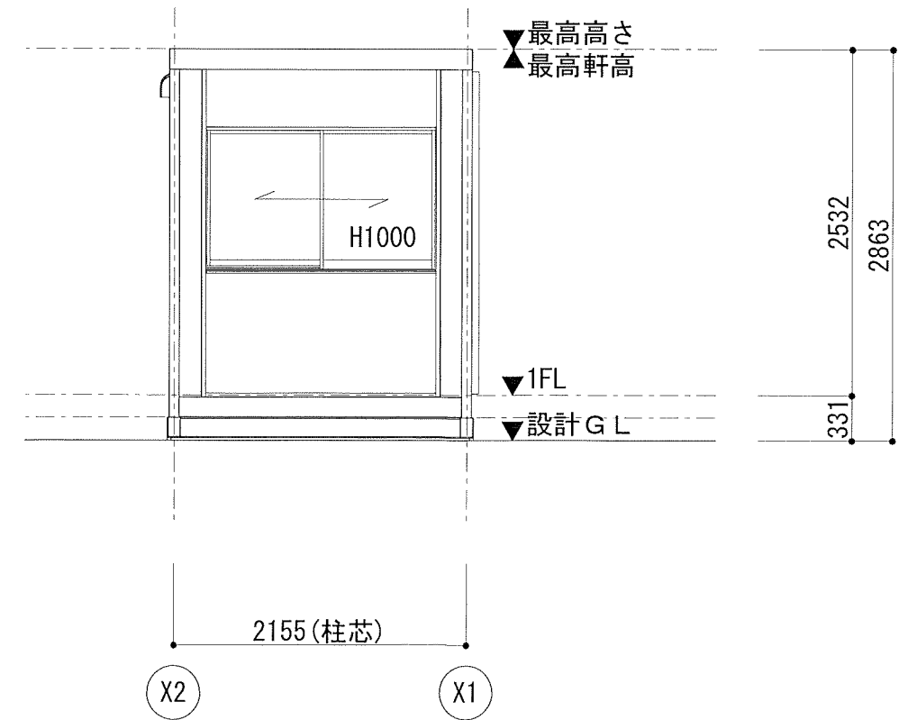
Y2通り立面図
