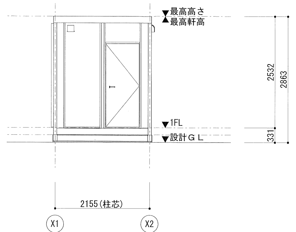
Y1通り立面図
