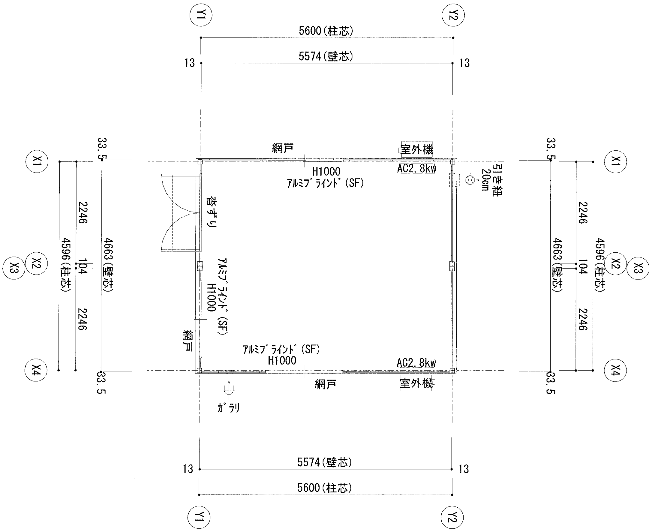
1階平面図
