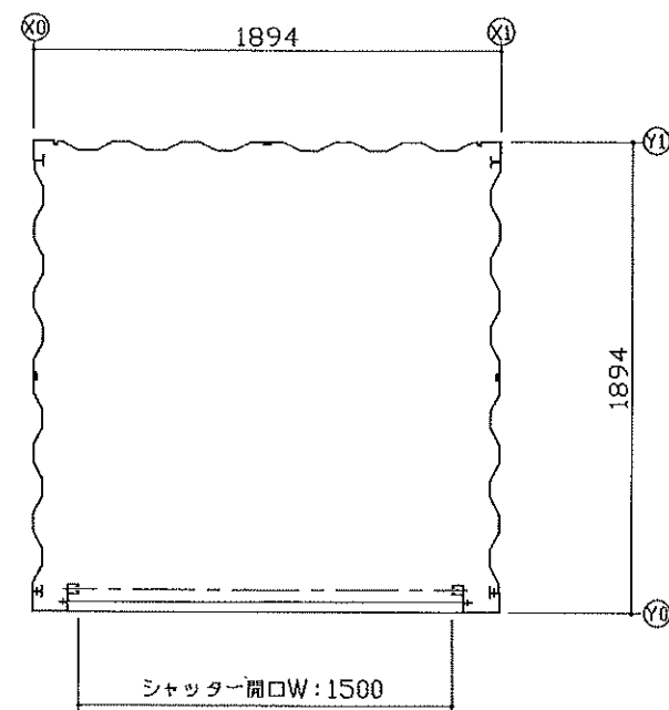
平面図
