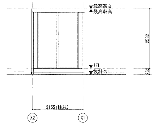
Y2通り立面図
