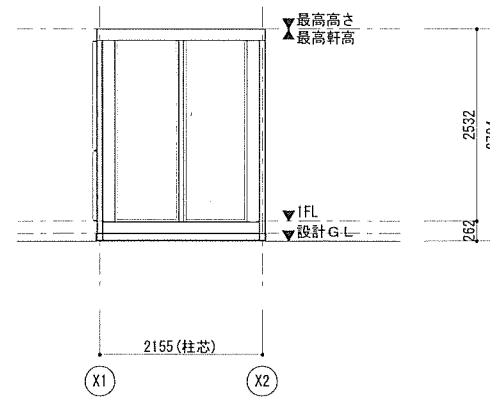
Y1通り立面図
