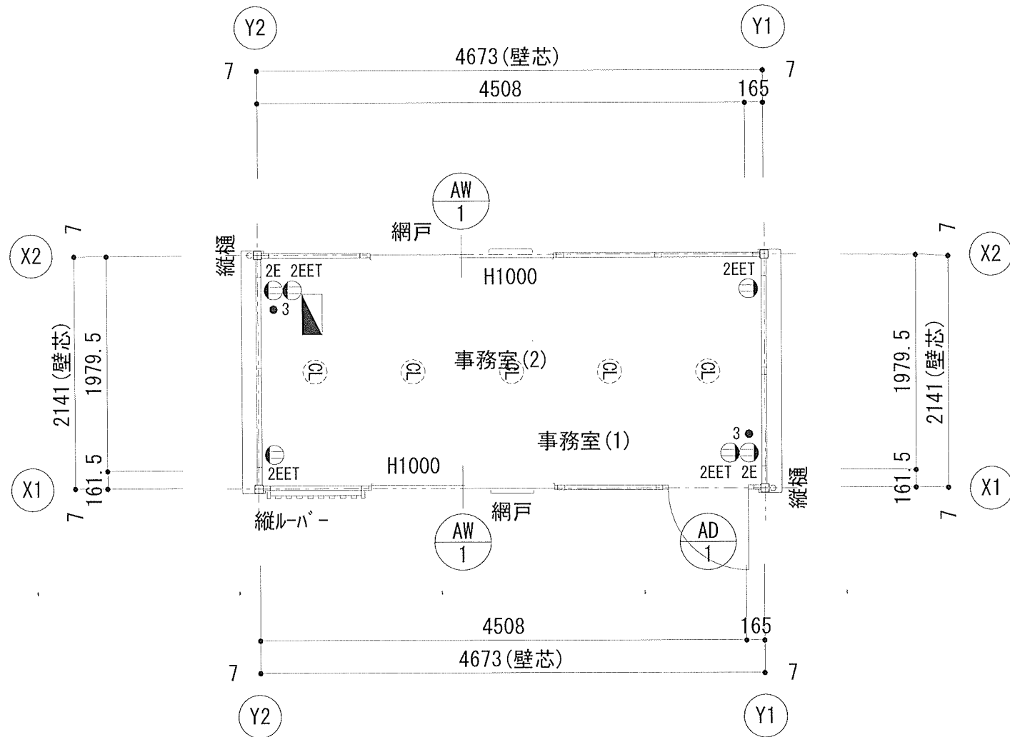
1階平面図
