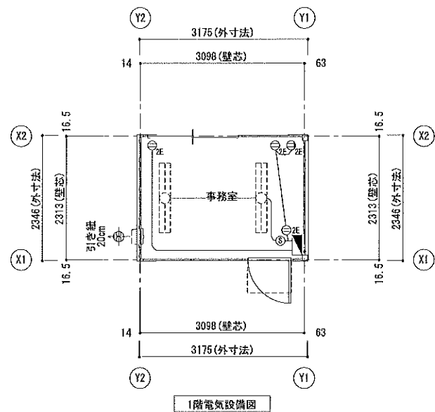
1階電気設備図
