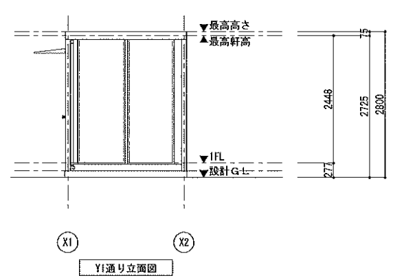
Y1通り立面図
