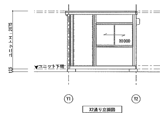
X2通り立面図
