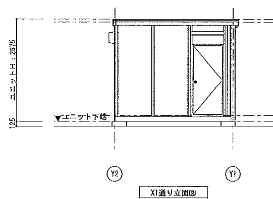
X1通り立面図
