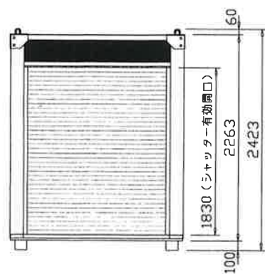
正面図
