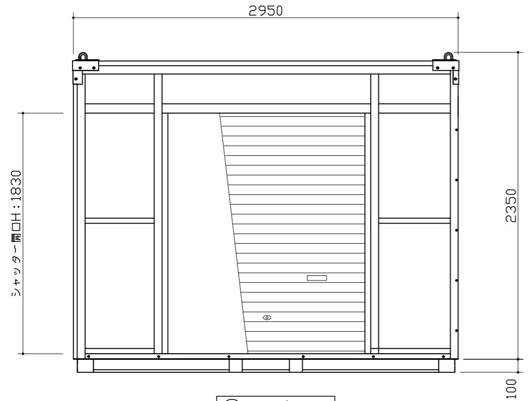
Y0 通り立面図
