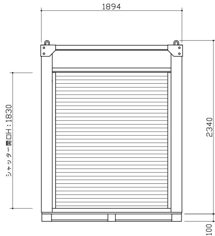
Y0通り立面図
