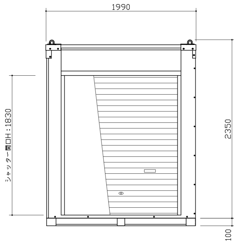
⑫通り立面図
