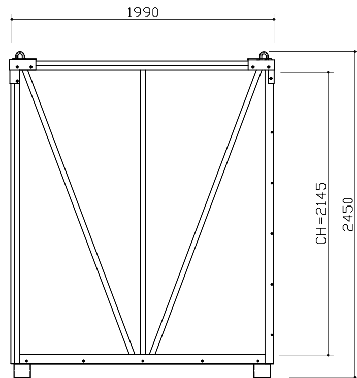
X1 通り立面図
