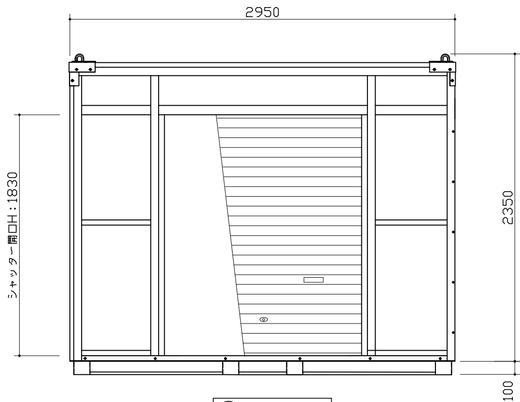
Y0 通り立面図
