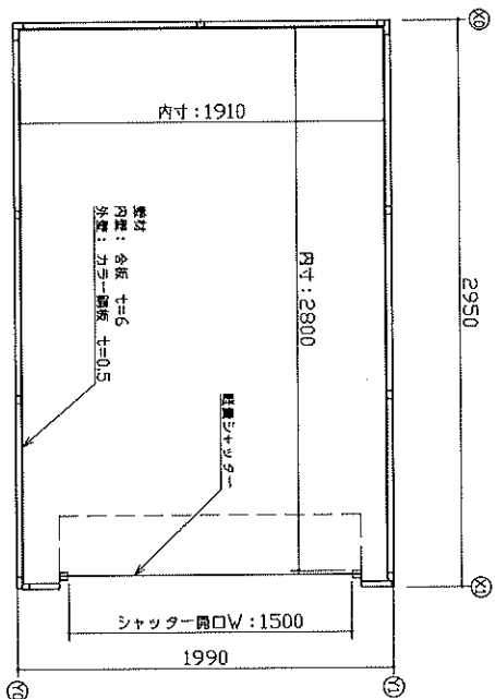
平面図
