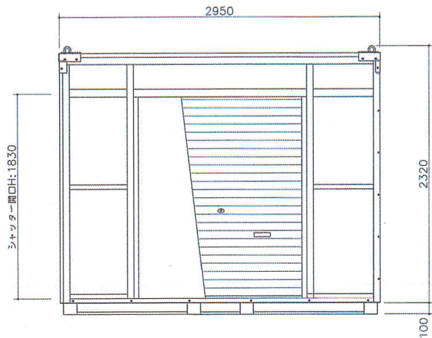
Y0通り立面図
