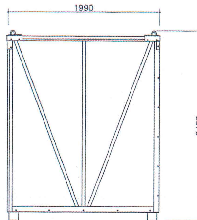
X1通り立面図
