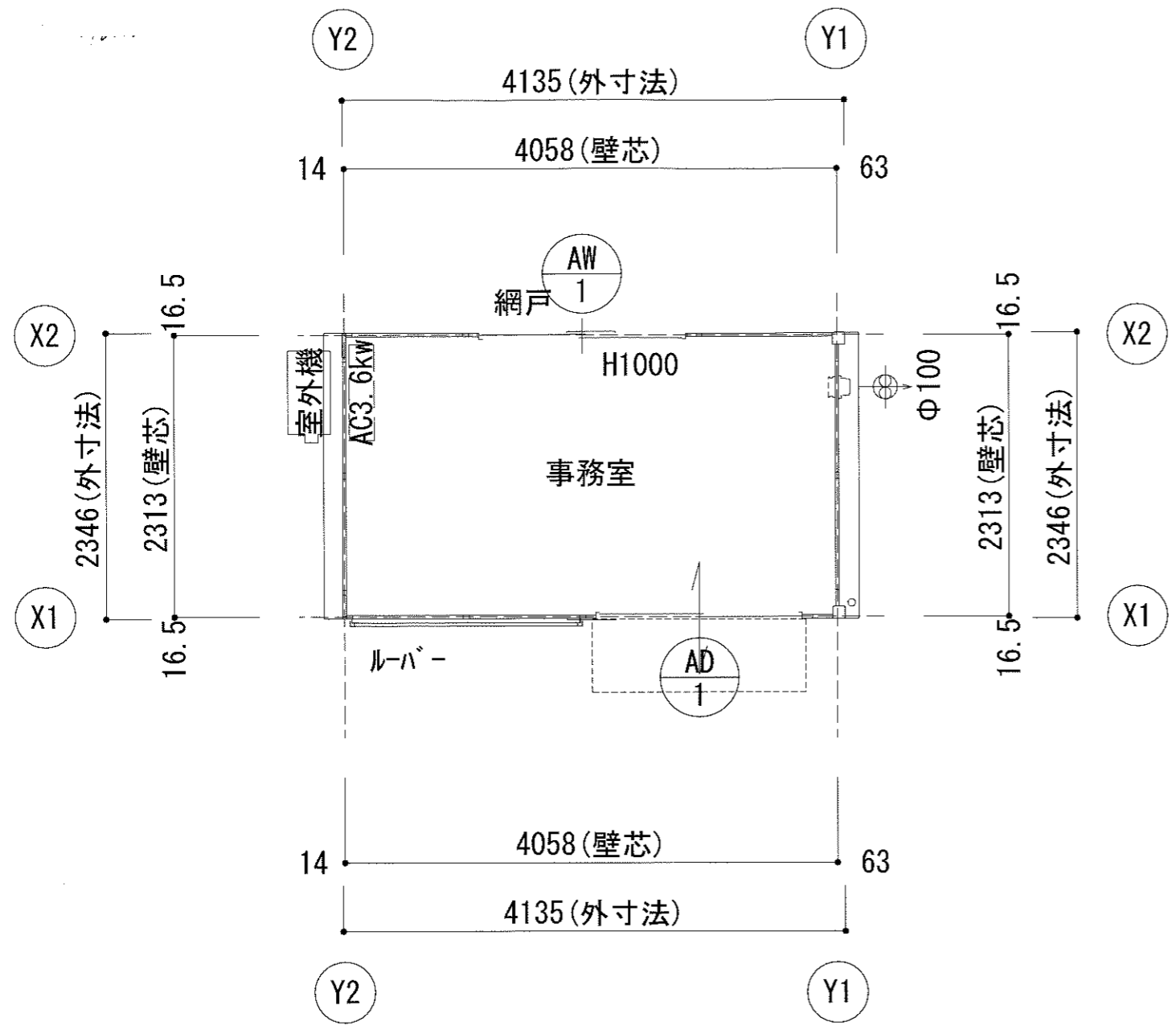
1階平面図
