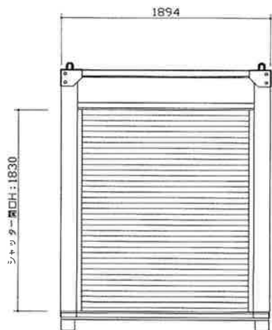
X10通り立面図
