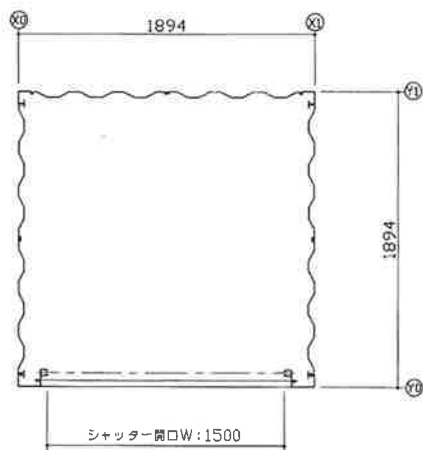
シャッター開口W:1500 平面図
