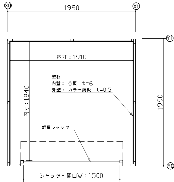
平面図
