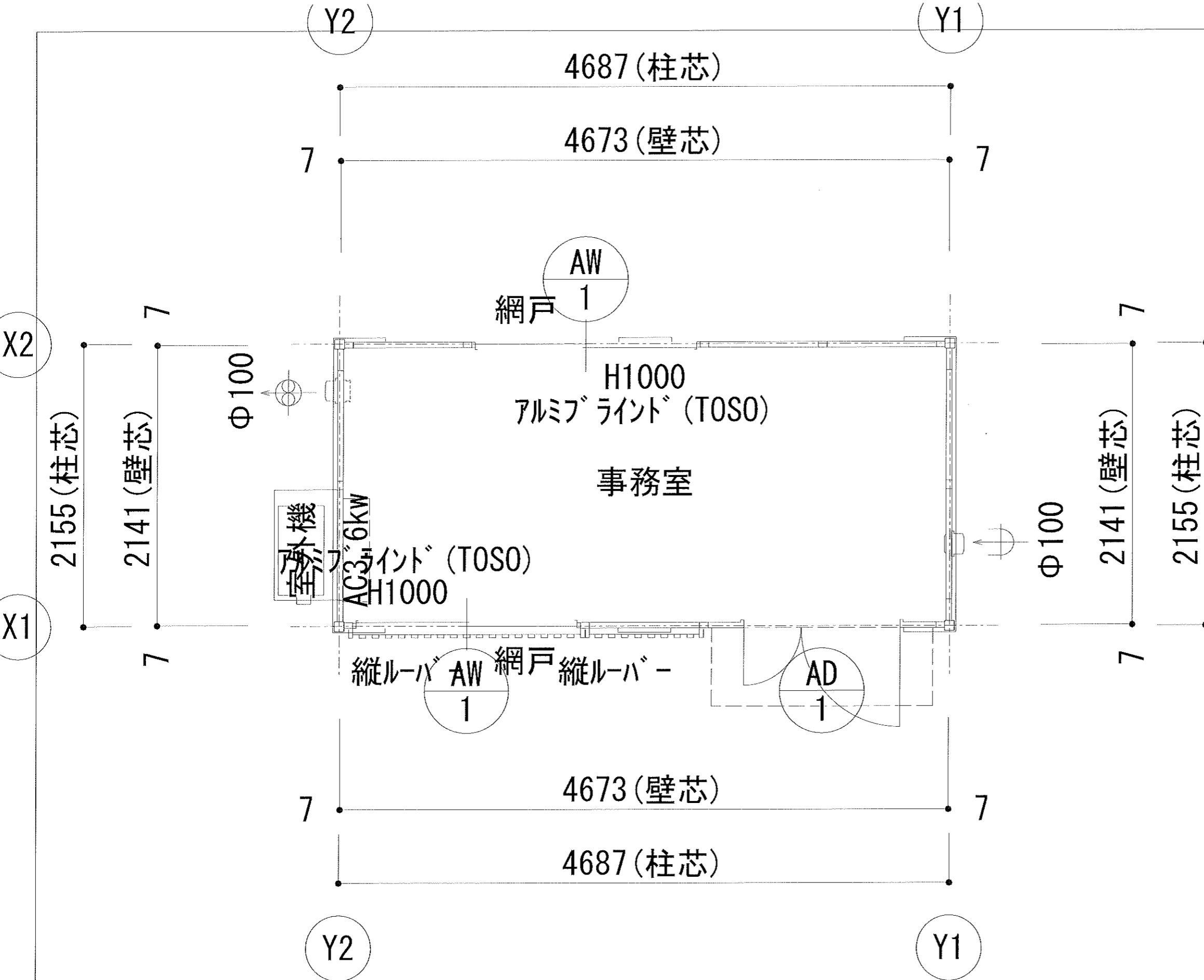
1階平面図
