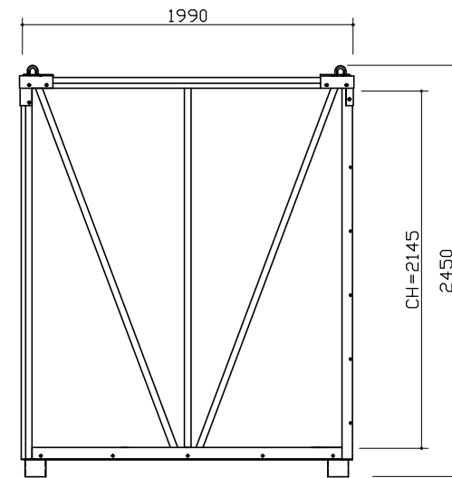
X1通り立面図
