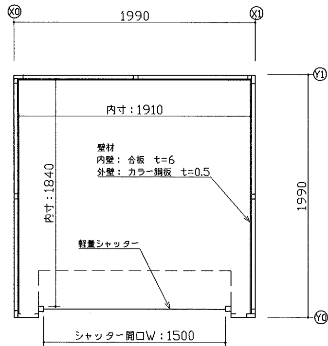
平面図
