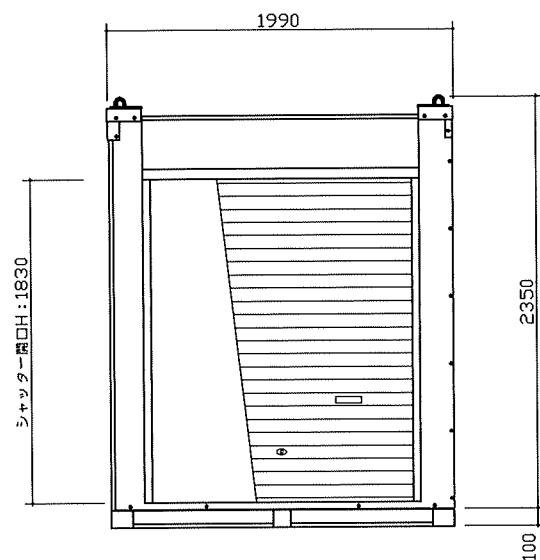
Y0 通り立面図
