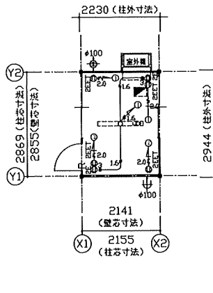
電気配線図
