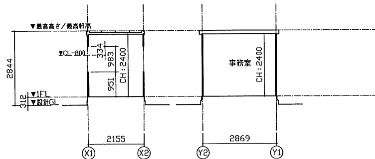
A-A断面図
