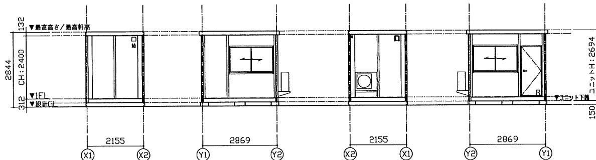
Y1通り立面図
