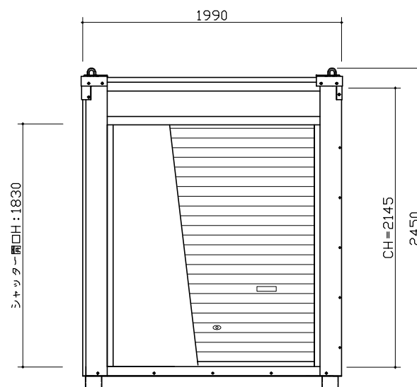
X1通り立面図
