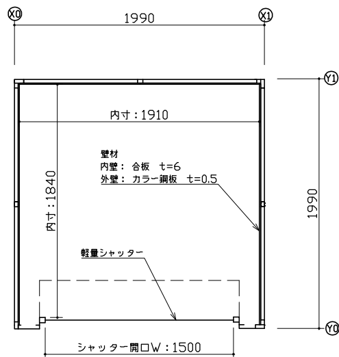
平面図
