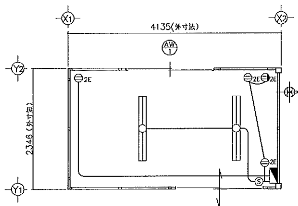
平面図
