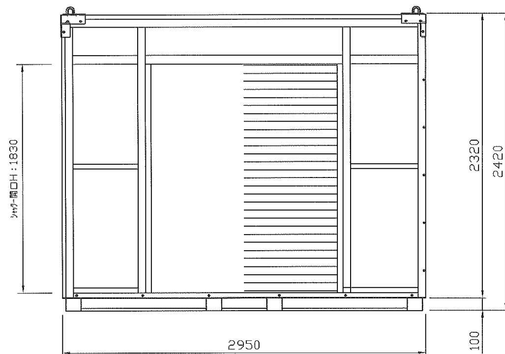
Y0通り立面図
