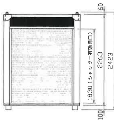
正面図
