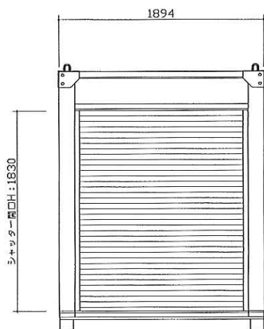
Y0通り立面図
