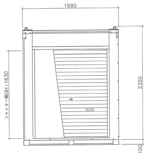
Y0通り立面図
