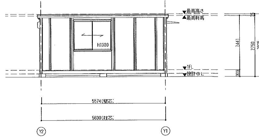
X1通り立面図
