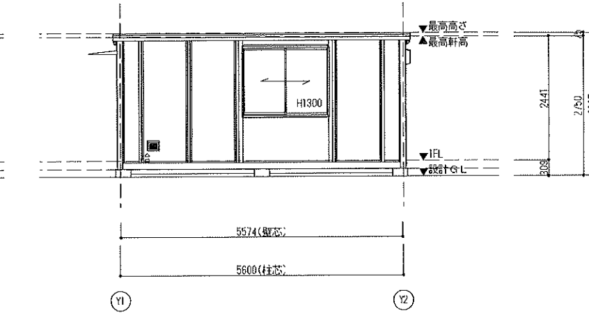
X2通り立面図
