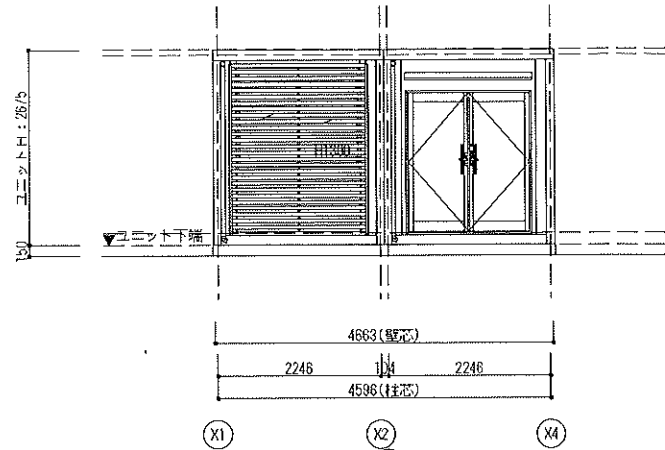
Y1通り立面図
