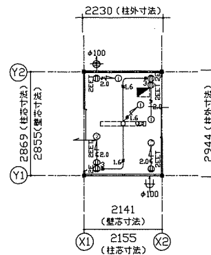
電気配線図
