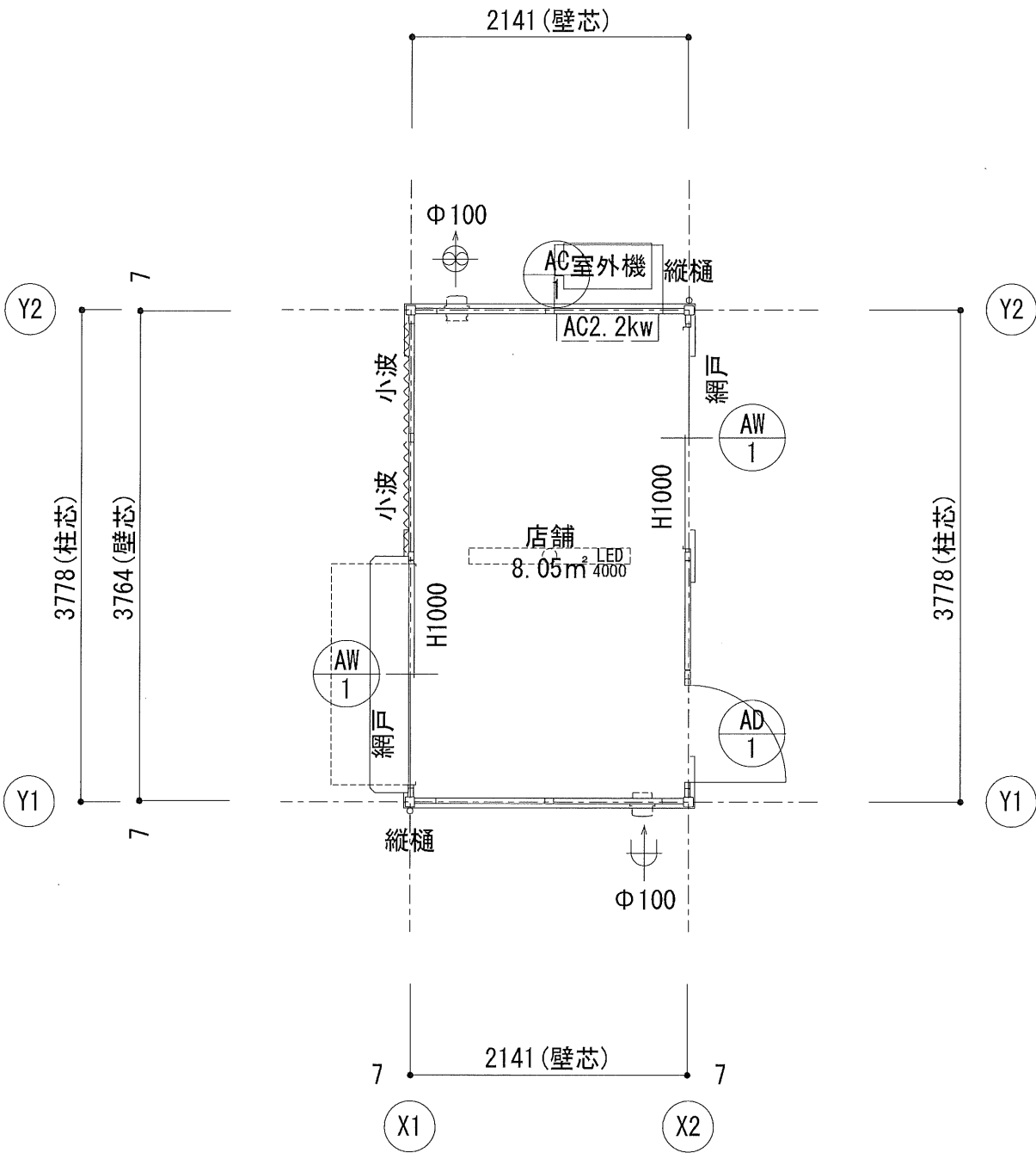
1階平面図
