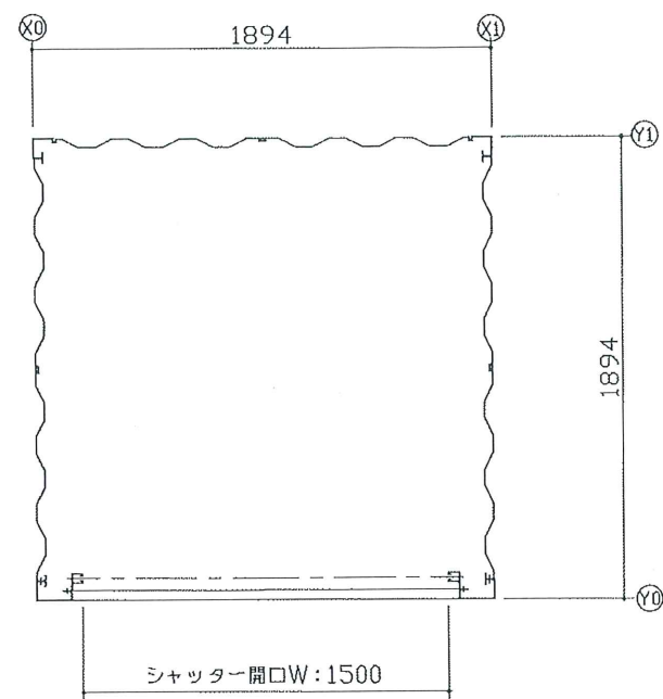
平面図
