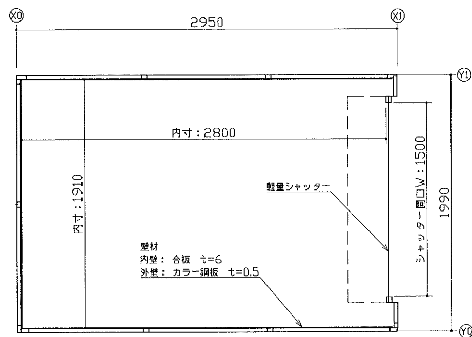
平面図
