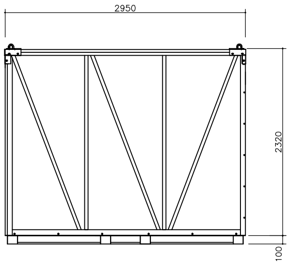
⑬通り立面図
