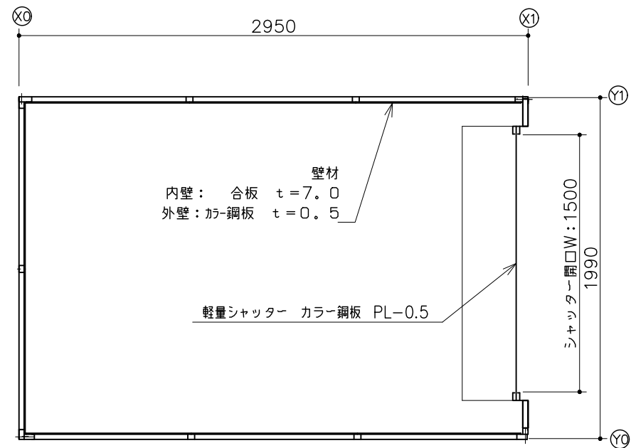
平面図
