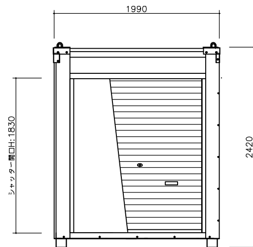
⑩通り立面図
