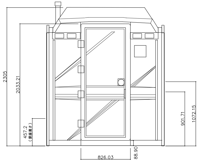
立面図
