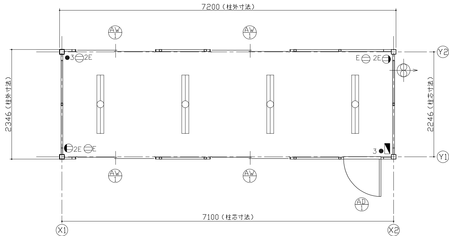
平面図
