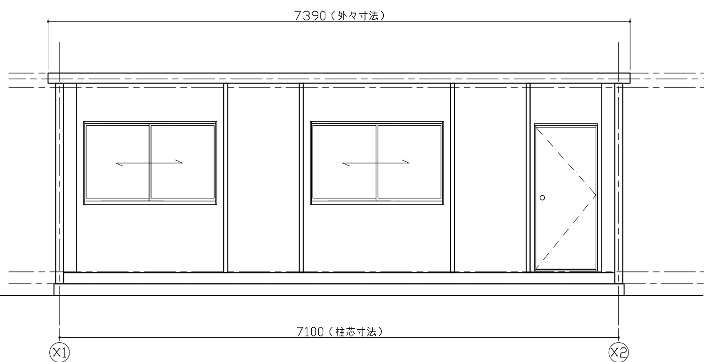
(Y1) 通り立面図
