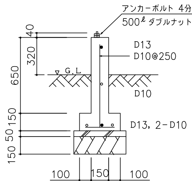
基礎断面図 S=1/20
