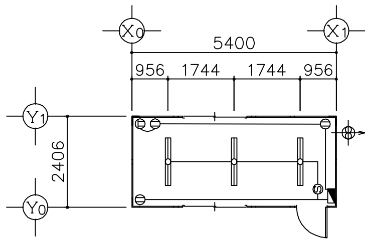
平面図 S=1/100
